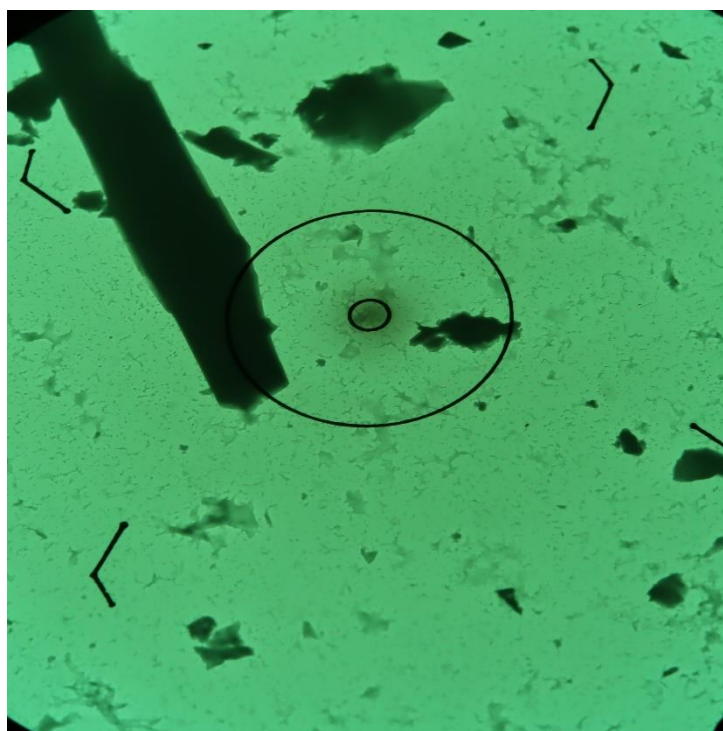
Obr. 1 Mikrofoto TEM vz. 16956/68, úlomky horniny. Zvětšeno 2500x, průměr vnitřního terče je 1,9 \mu\text{m} .
