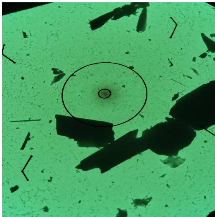
Obr. 1 Mikrofoto TEM vz. 16979/71, úlomky horniny. Zvětšeno 2500x, průměr vnitřního terče je 1,9 \mu\text{m} .
