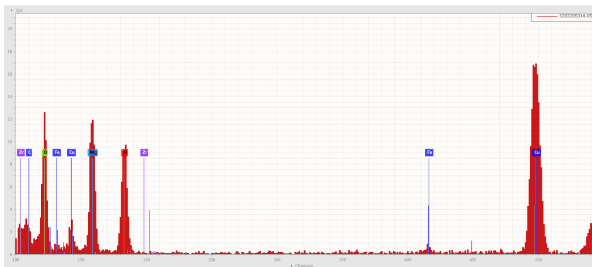
Obr. 3 EDS spektrum chryzotilového azbestového vlákna, vz. 16903/52.
