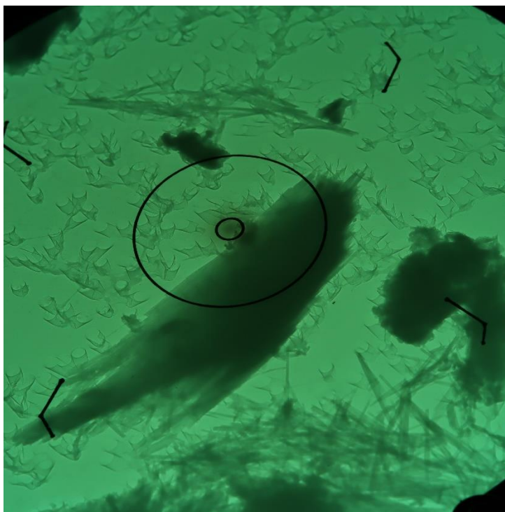
Obr. 2 Mikrofoto TEM vz. 16903/52, azbestová vlákna. Zvětšeno 13500x, průměr vnitřního terče je 0,4 \mu\text{m} .
