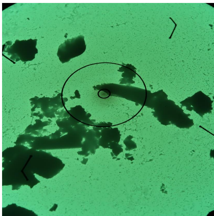
Obr. 1 Mikrofoto TEM vz. 16992/56, úlomky horniny. Zvětšeno 2500x, průměr vnitřního terče je 1,9 \mu\text{m} .
