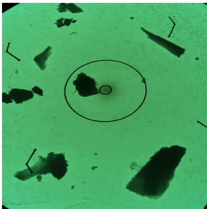
Obr. 1 Mikrofoto TEM vz. 16943/40, úlomky horniny. Zvětšeno 2500x, průměr vnitřního terče je 1,9 \mu\text{m} .
