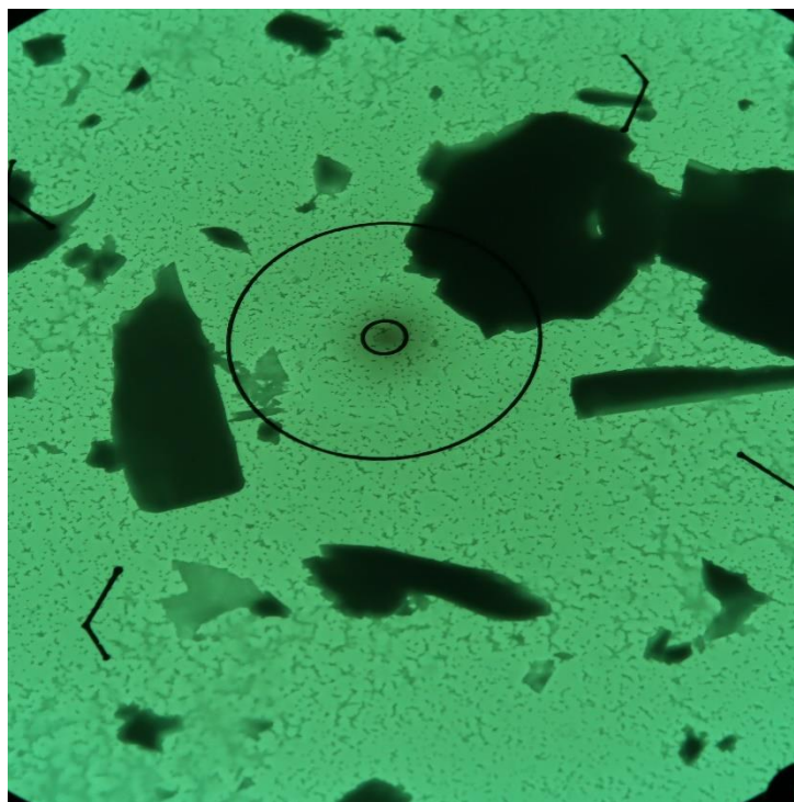
Obr. 1 Mikrofoto TEM vz. 17024/47, úlomky horniny. Zvětšeno 2500x, průměr vnitřního terče je 1,9 \mu\text{m} .
