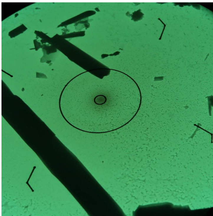
Obr. 1 Mikrofoto TEM vz. 16882/65, úlomky horniny. Zvětšeno 2500x, průměr vnitřního terče je 1,9 \mu\text{m} .
