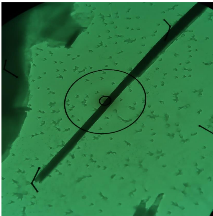
Obr. 2 Mikrofoto TEM vz. 16882/65, azbestové vlákno. Zvětšeno 13500x, průměr vnitřního terče je 0,4 \mu\text{m} .
