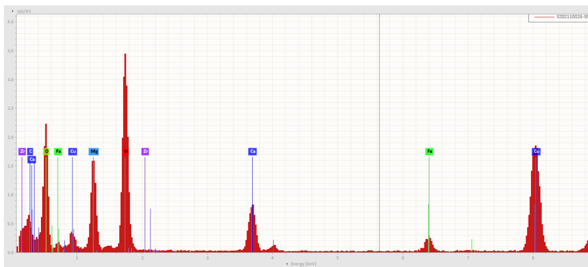
Obr. 3 EDS spektrum aktinolitového azbestového vlákna, vz. 16882/65.
