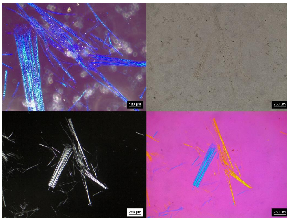
Obr. 1 Mikrofoto OPM vz. 16895/30, azbestová vlákna (ve směru čtení postupně: objektiv disperzního barvení, rovnoběžné polarizátory, zkřížené polarizátory, zkřížené polarizátory s destičkou fázového posunu 530 nm).
