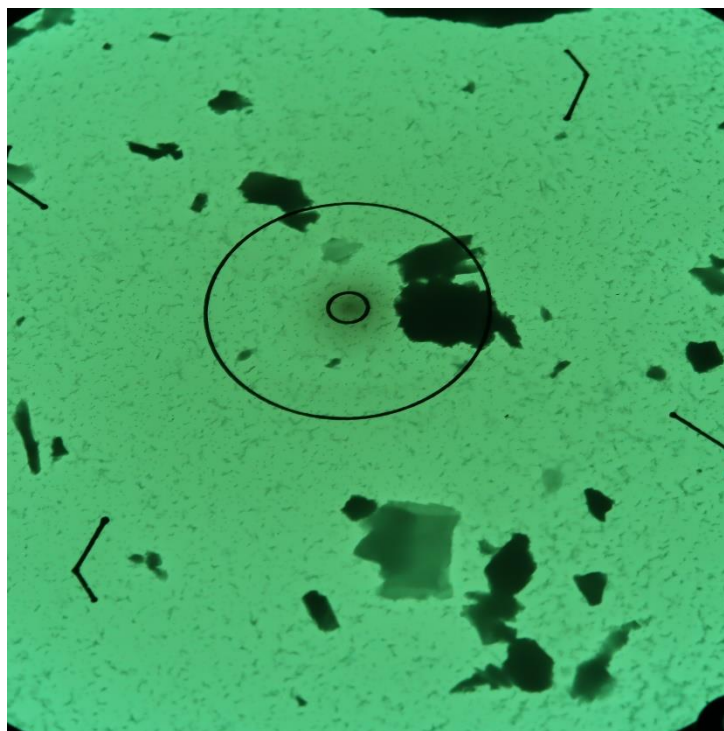
Obr. 1 Mikrofoto TEM vz. 17016/41, úlomky horniny. Zvětšeno 2500x, průměr vnitřního terče je 1,9 \mu\text{m} .
