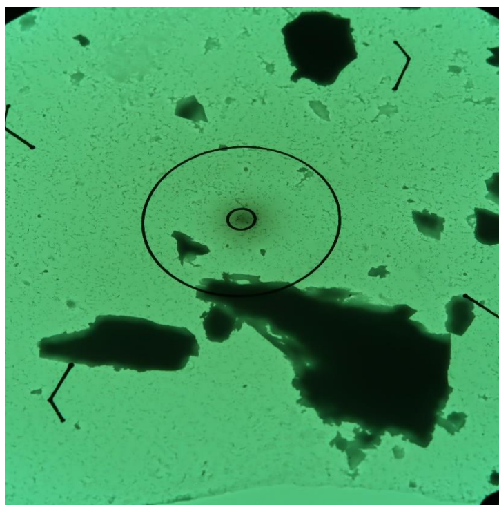
Obr. 1 Mikrofoto TEM vz. 16995/35, úlomky horniny. Zvětšeno 2500x, průměr vnitřního terče je 1,9 \mu\text{m} .
