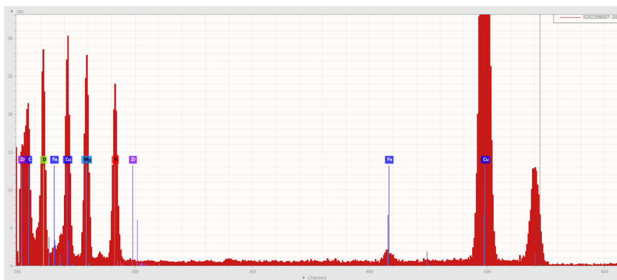
Obr. 3 EDS spektrum chryzotilového azbestového vlákna, vz. 17177/92.
