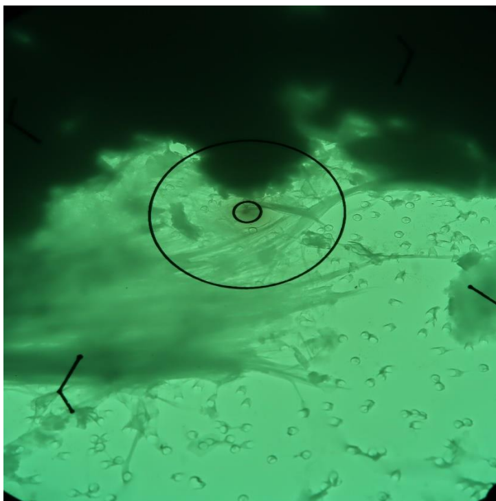
Obr. 2 Mikrofoto TEM vz. 17177/92, azbestová vlákna. Zvětšeno 13500x, průměr vnitřního terče je 0,4 \mu\text{m} .
