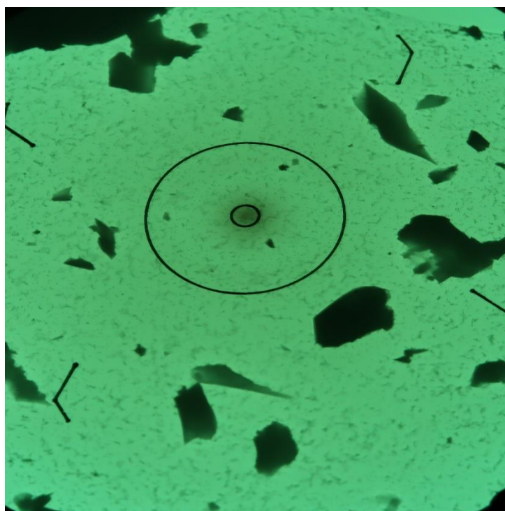
Obr. 1 Mikrofoto TEM vz. 17061/8, úlomky horniny. Zvětšeno 2500x, průměr vnitřního terče je 1,9 \mu\text{m} .
