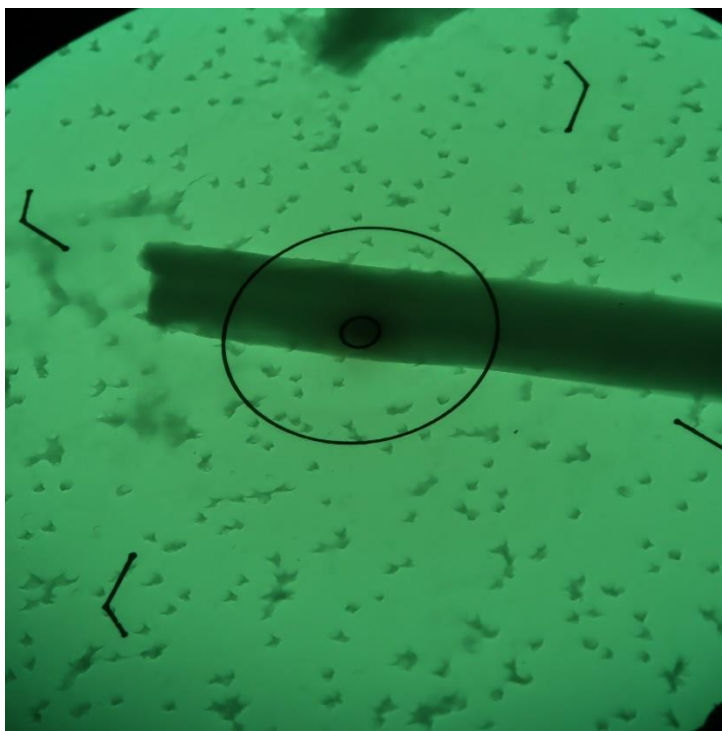
Obr. 2 Mikrofoto TEM vz. 16897/81, azbestové vlákno. Zvětšeno 13500x, průměr vnitřního terče je 0,4 \mu\text{m} .
