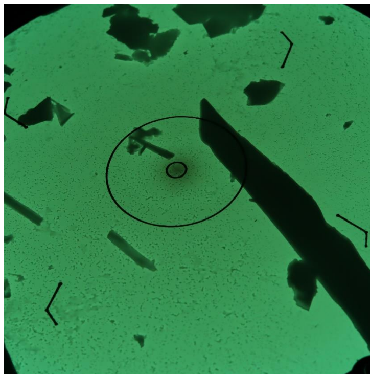
Obr. 1 Mikrofoto TEM vz. 16897/81, úlomky horniny. Zvětšeno 2500x, průměr vnitřního terče je 1,9 \mu\text{m} .
