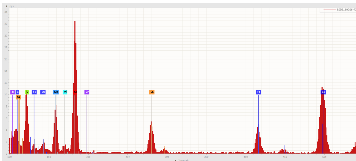
Obr. 3 EDS spektrum aktinolitového azbestového vlákna, vz. 16897/81.
