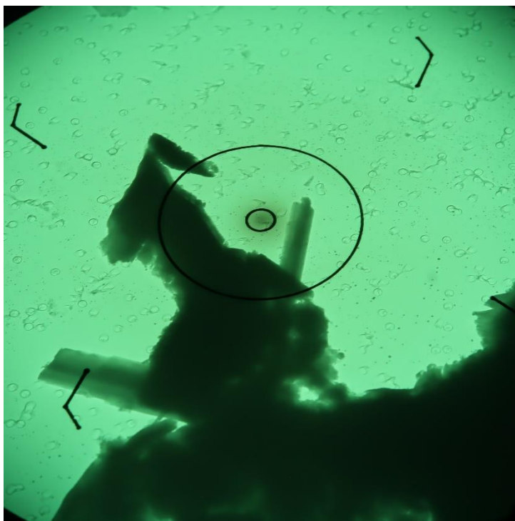
Obr. 2 Mikrofoto TEM vz. 17068/91, azbestová vlákna. Zvětšeno 13500x, průměr vnitřního terče je 0,4 \mu\text{m} .
