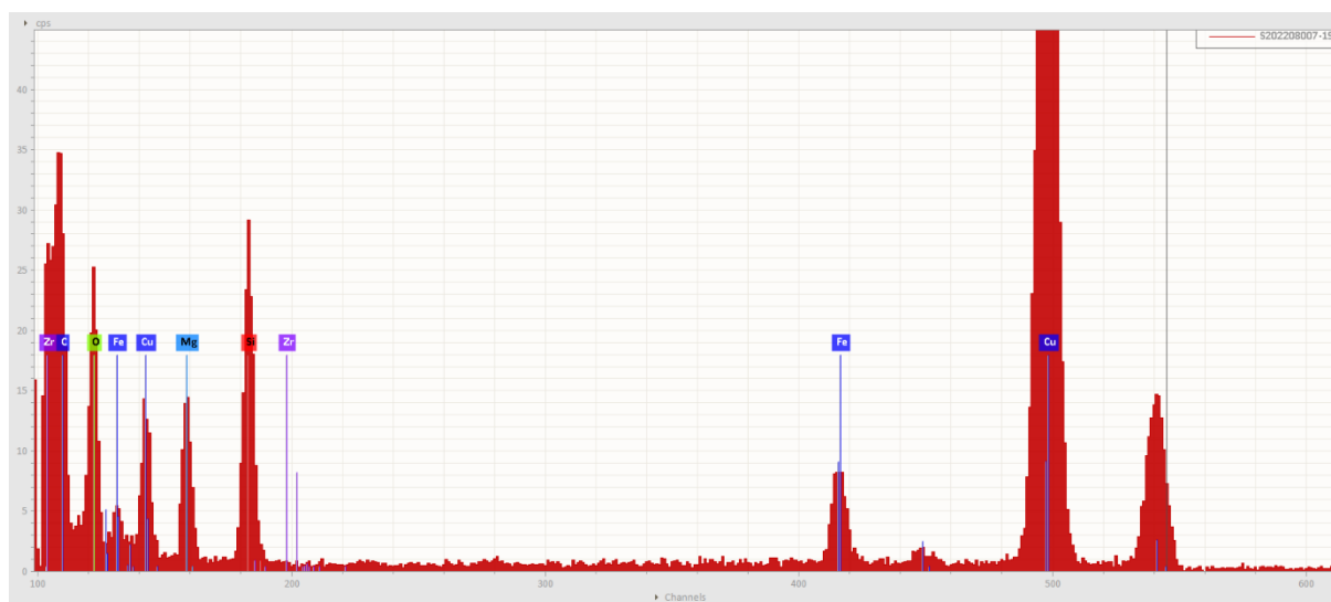
Obr. 3 EDS spektrum antofylitového azbestového vlákna, vz. 17068/91.
