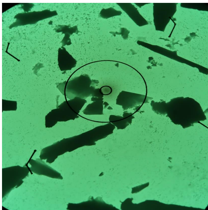
Obr. 1 Mikrofoto TEM vz. 16955/76, úlomky horniny. Zvětšeno 2500x, průměr vnitřního terče je 1,9 \mu\text{m} .
