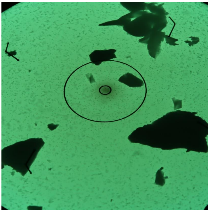
Obr. 1 Mikrofoto TEM vz. 17026/25, úlomky horniny. Zvětšeno 2500x, průměr vnitřního terče je 1,9 \mu\text{m} .
