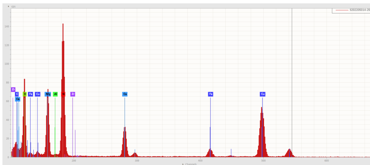
Obr. 3 EDS spektrum tremolitového azbestového vlákna, vz. 16978/67.
