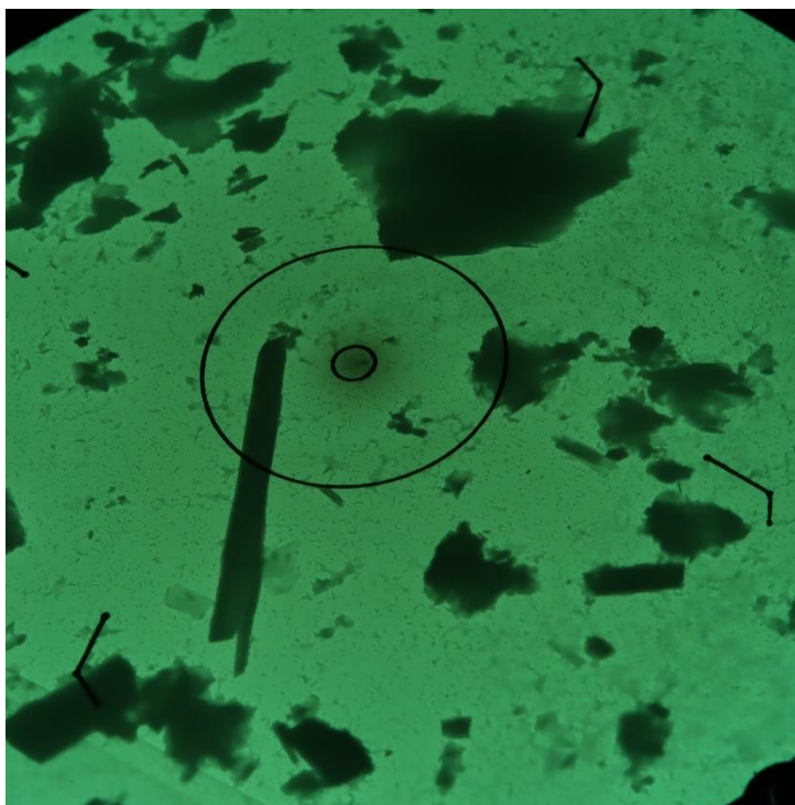
Obr. 1 Mikrofoto TEM vz. 16978/67, úlomky horniny. Zvětšeno 2500x, průměr vnitřního terče je 1,9 μm.
