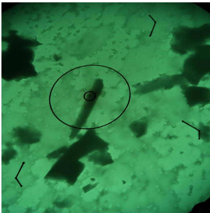
Obr. 2 Mikrofoto TEM vz. 16998/10, azbestové vlákno. Zvětšeno 13500x, průměr vnitřního terče je 0,4 \mu\text{m} .
