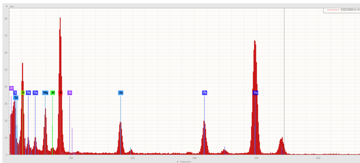
Obr. 3 EDS spektrum aktinolitového azbestového vlákna, vz. 16998/10.
