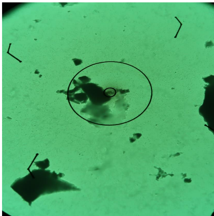
Obr. 1 Mikrofoto TEM vz. 16945/45, úlomky horniny. Zvětšeno 2500x, průměr vnitřního terče je 1,9 \mu\text{m} .
