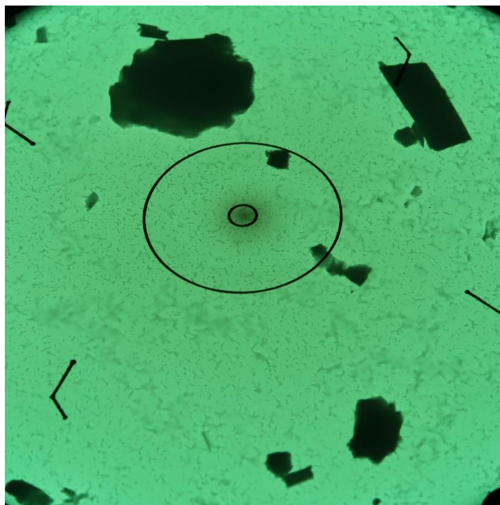
Obr. 1 Mikrofoto TEM vz. 17014/44, úlomky horniny. Zvětšeno 2500x, průměr vnitřního terče je 1,9 \mu\text{m} .
