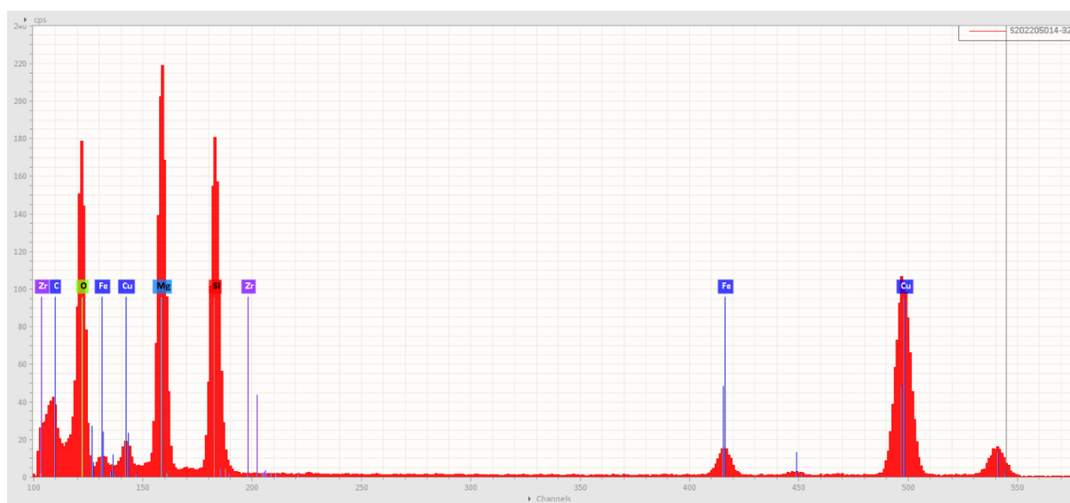
Obr. 3 EDS spektrum chryzotilového azbestového vlákna, vz. 16999/61.
