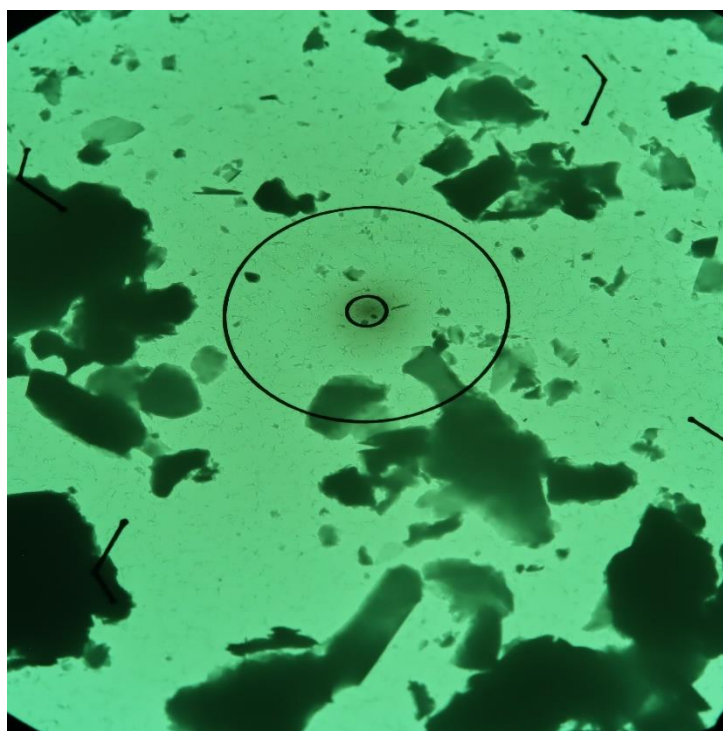
Obr. 1 Mikrofoto TEM vz. 16898/86, úlomky horniny. Zvětšeno 2500x, průměr vnitřního terče je 1,9 \mu\text{m} .
